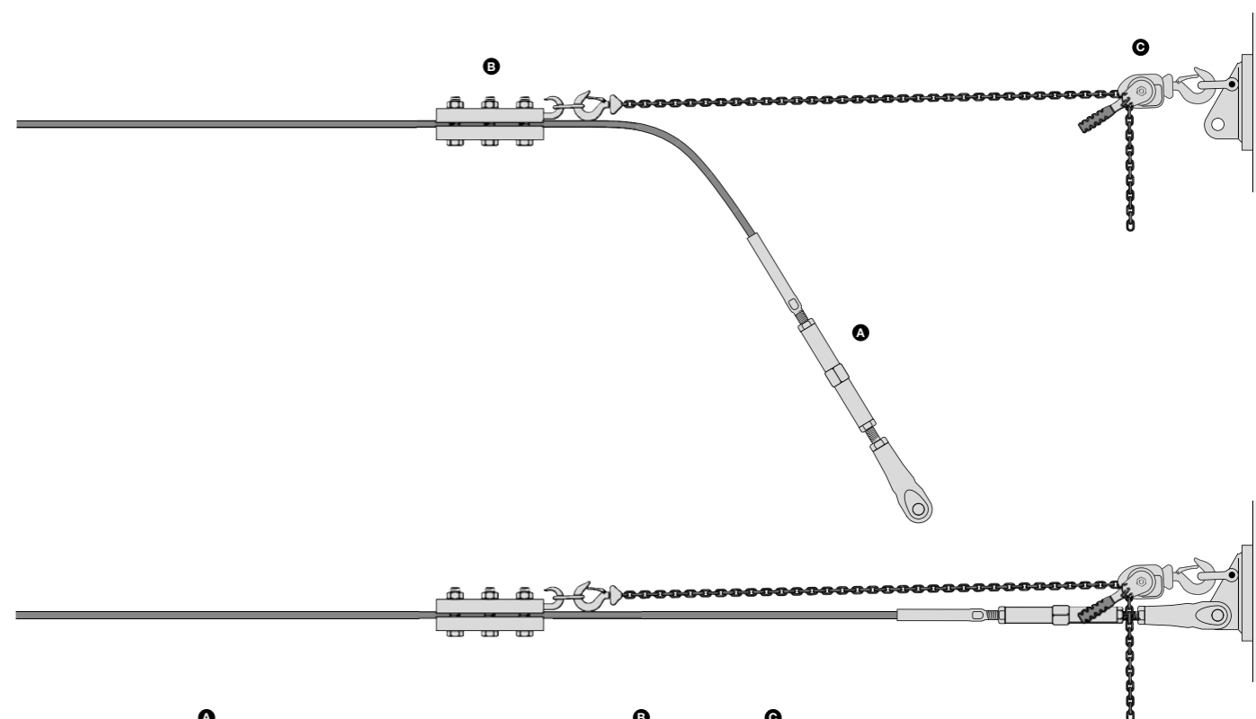
A Seilvorspannung / Prétension des câbles / Rope pre-stretching Seil mit Spannschloss mit Gabel Forte rund verpresst / Câble avec tuyau de serrage avec chape Forte serti rond / Rope with turnbuckle with clevis Forte round swaged B Abspannklemme / Serre-câble / Straining clamp C Kettenzug / Palan à chaînes / Chain hoist
